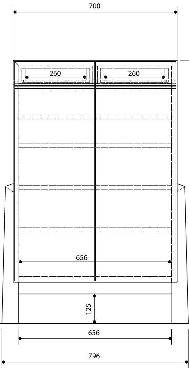
【正面】
