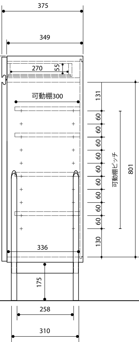
【側面】
